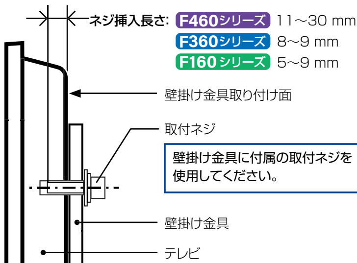
取り付け部断面図の一例
