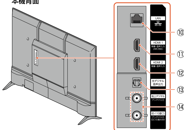
本機背面
